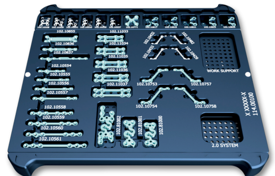
Conjunto 109.40074 Estojo Ortognático
