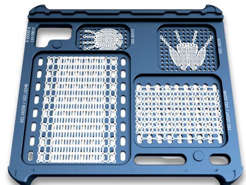
Conjunto 109.40081 Estorjo Trauma 1,5
