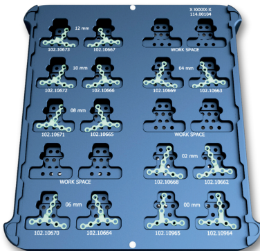
Conjunto 109.40078 Estojo Lefort 2,0 5x3
