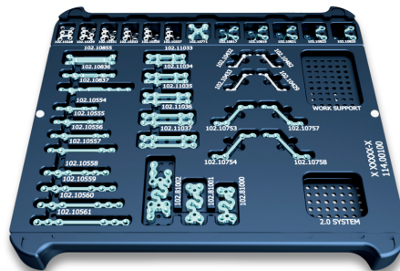
Conjunto 109.40074 Estorjo Ortognática
